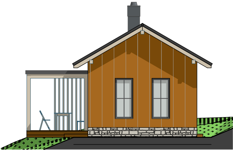
Pohled severní 1:100
