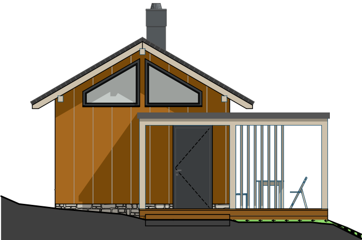
Pohled severní 1:100
